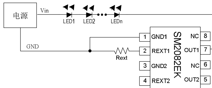
图 2. SM2082EK 应用电路原理图
