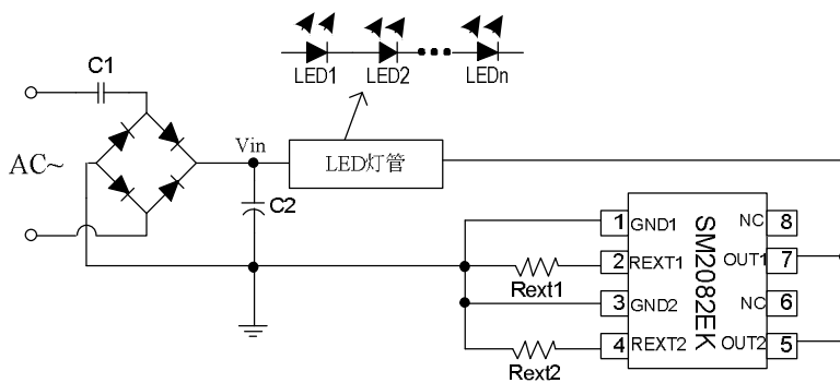
图 3. SM2082EK 典型应用电路—交流电源输入
