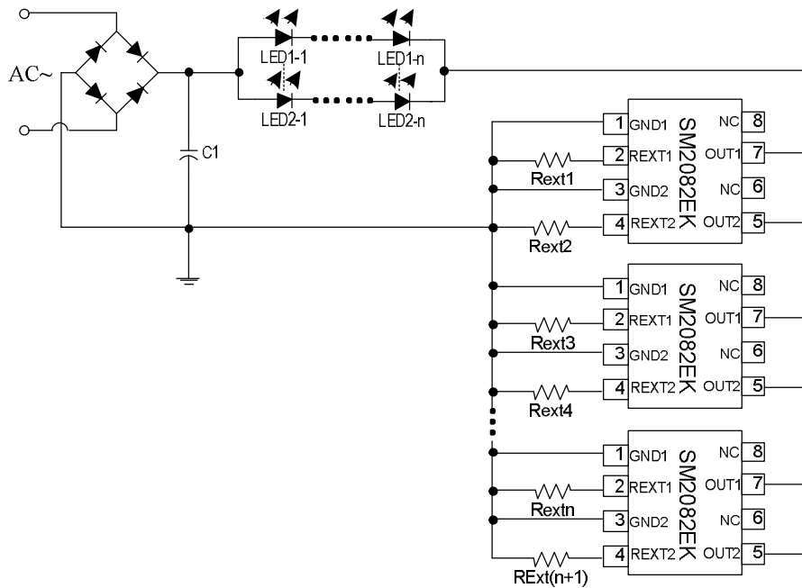
图 4. SM2082EK 并联应用电路原理图
