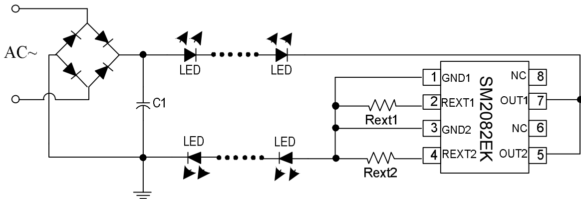
图 5. SM2082EK 串接 LED 灯管中
