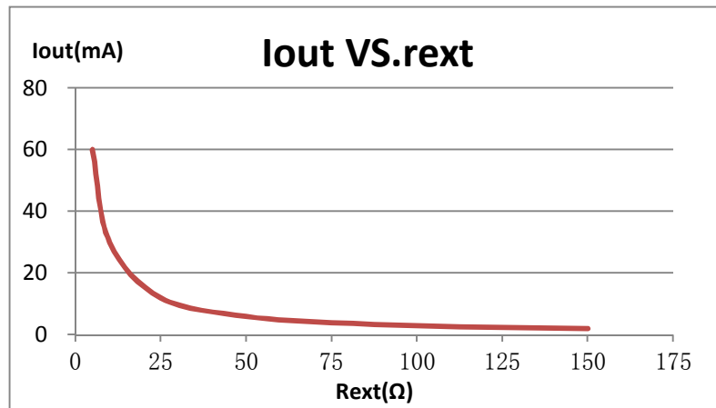
图 1. SM2082EK 输出电流与 Rext 电阻关系曲线
