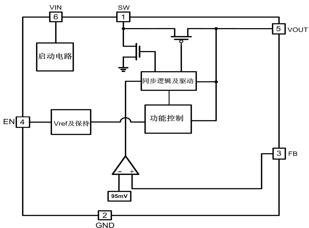
图 2. 内部框图
